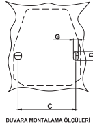
DUVARA MONTALAMA ÖLÇÜLERİ
