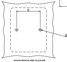
DUVAR MONTAJI ÖLÇÜLERİ
